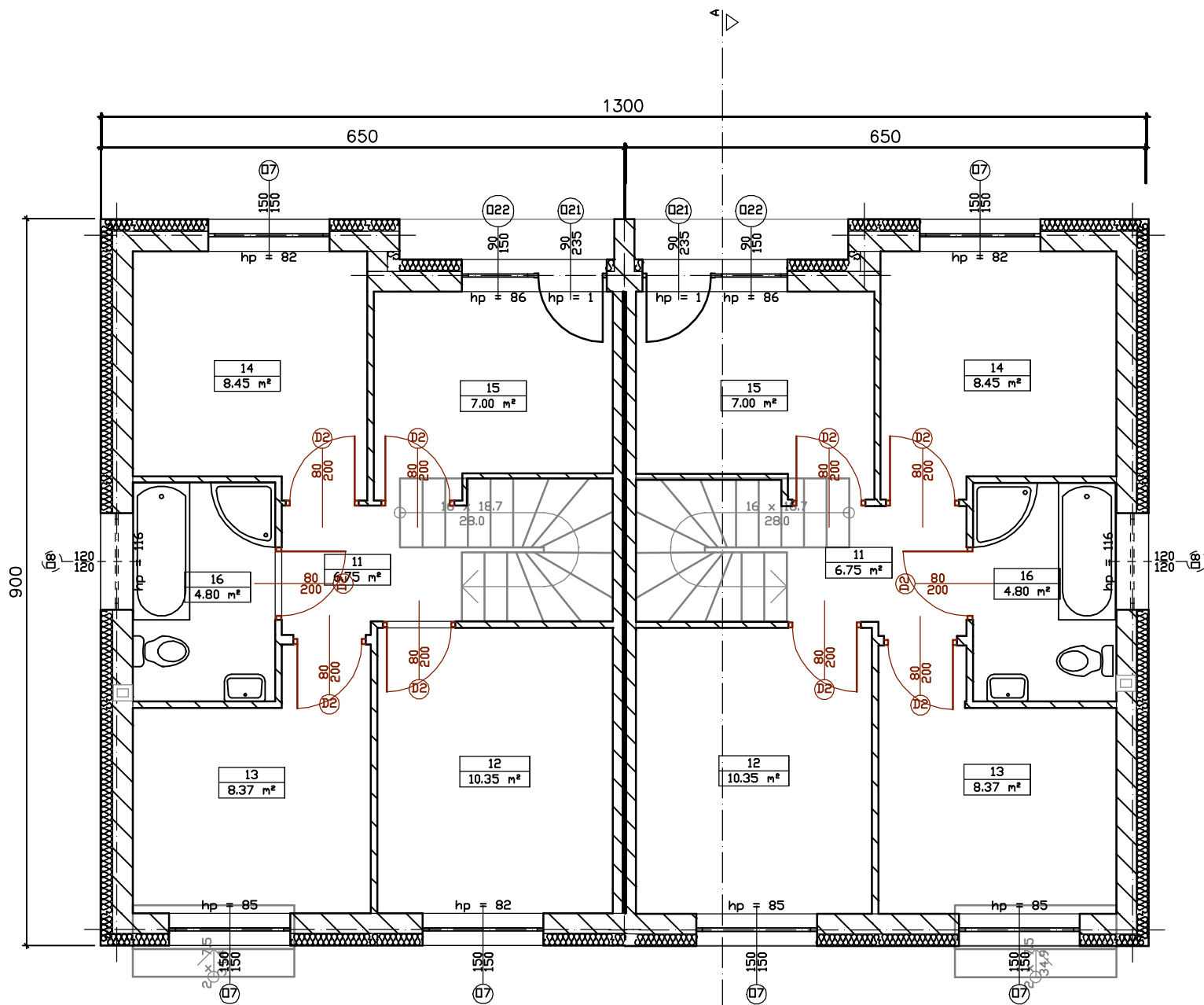
RZUT PIĘTRA
